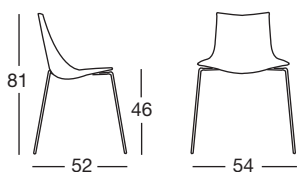
Struttura a 4 gambe 4-leg frame Art. 2273
